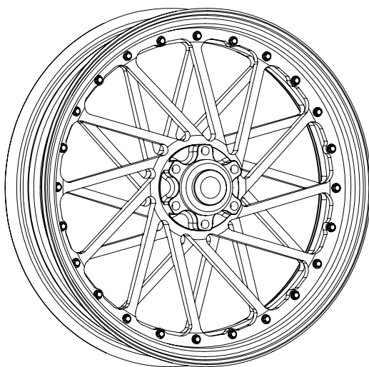
外圈螺絲:24個
